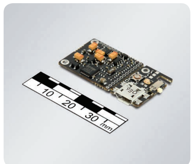
Цифровой диктофон ПАПИРУС-МИКРО (плата)
